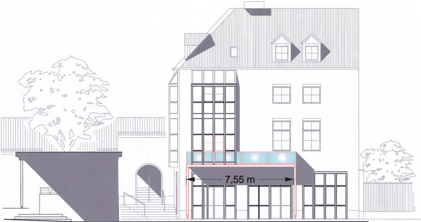
Nordost-Ansicht
