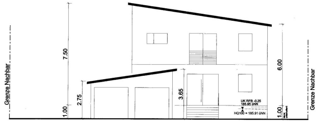
Ansicht M 1:100
