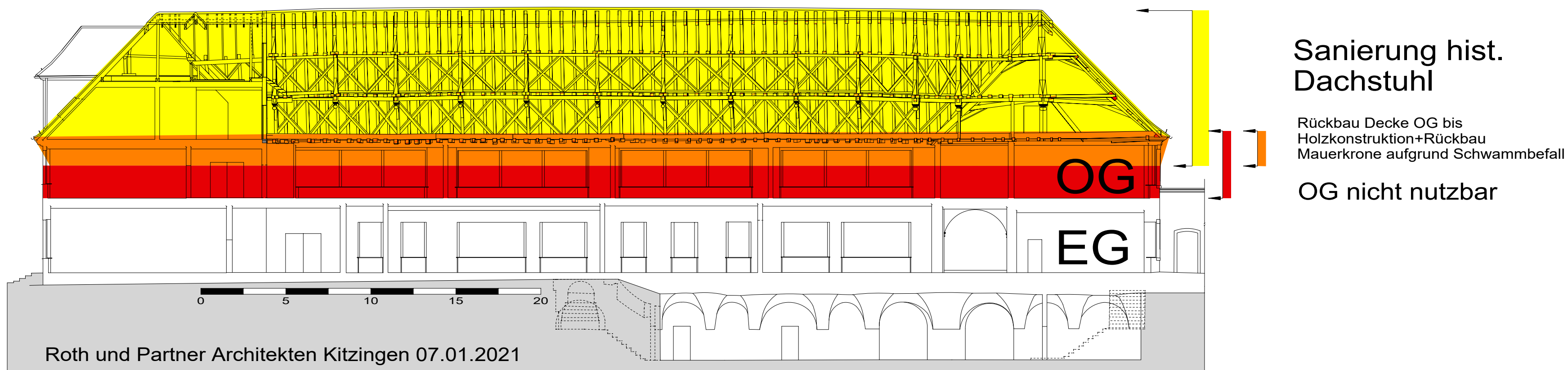
Friedrich Bernbeck Schule Kitzingen Längsschnitt 2
