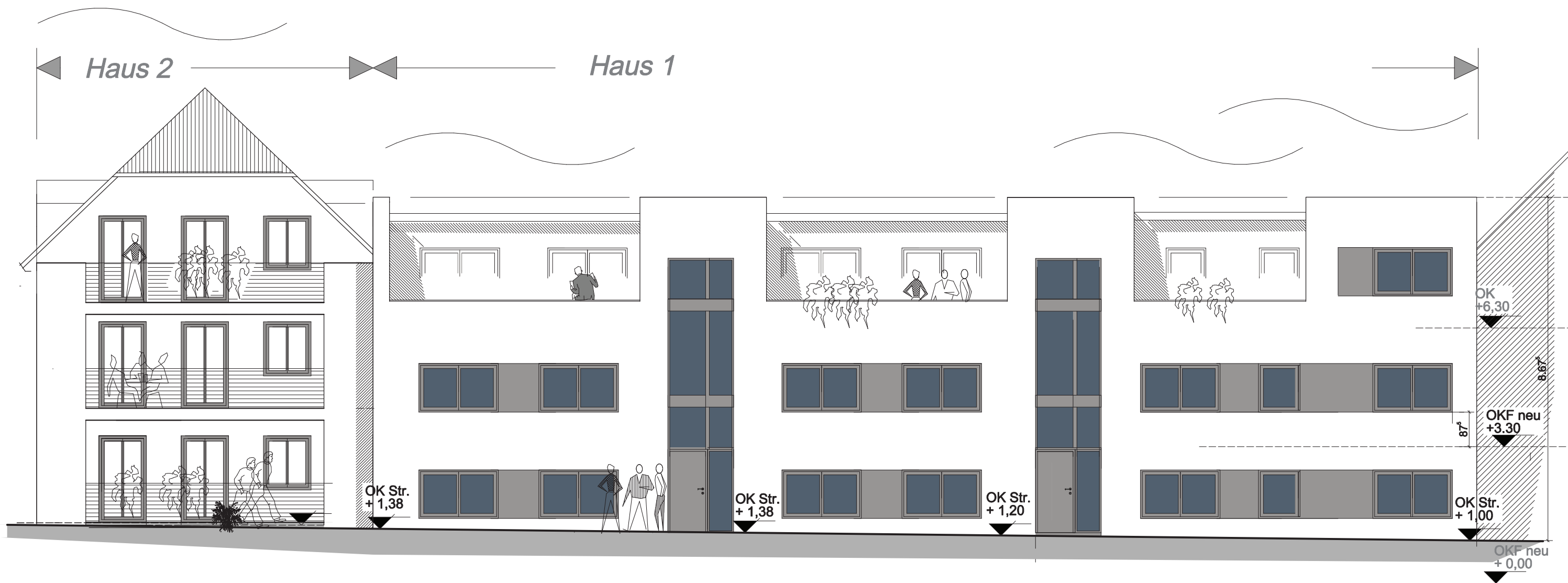
Nord-West Ansicht
